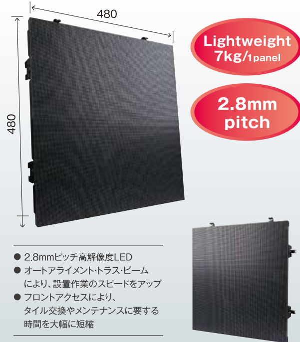
■ i-max Light 2.8 LEDスクリーン / 1パネルあたりの寸法図 (単位:mm)
