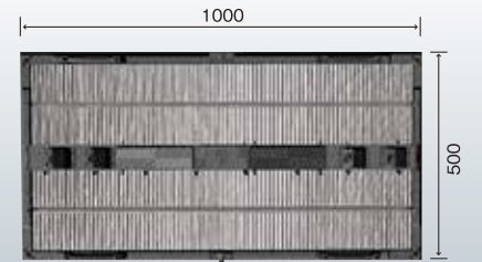
■ i-max Light 10w-m3 LEDスクリーン (単位:mm) / 1パネルあたりの寸法図
