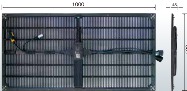
■ i-max Light 10w LEDスクリーン/1パネルあたりの寸法図 (単位:mm)
